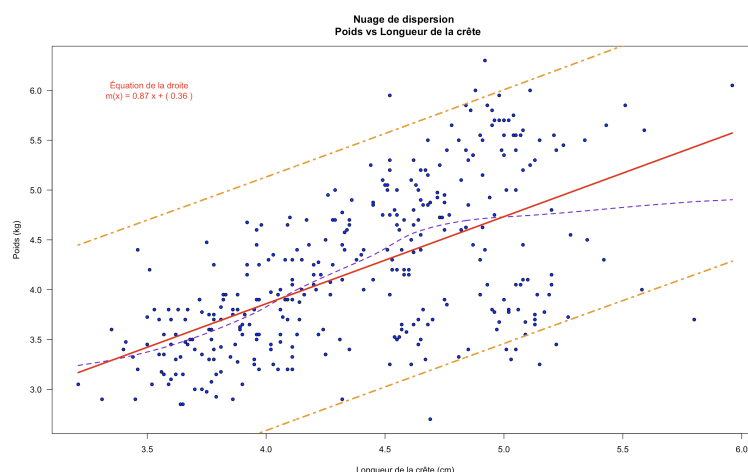
Fig. 3. Le poids des manchots en fonction de la longueur de la crête supérieure du bec
