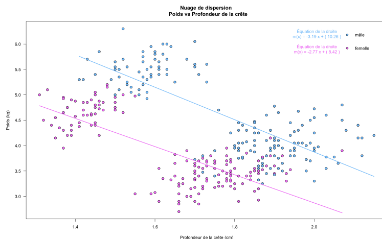
Fig. 7. Le poids des manchots en fonction de la profondeur de la crête supérieur du bec, selon le sexe
